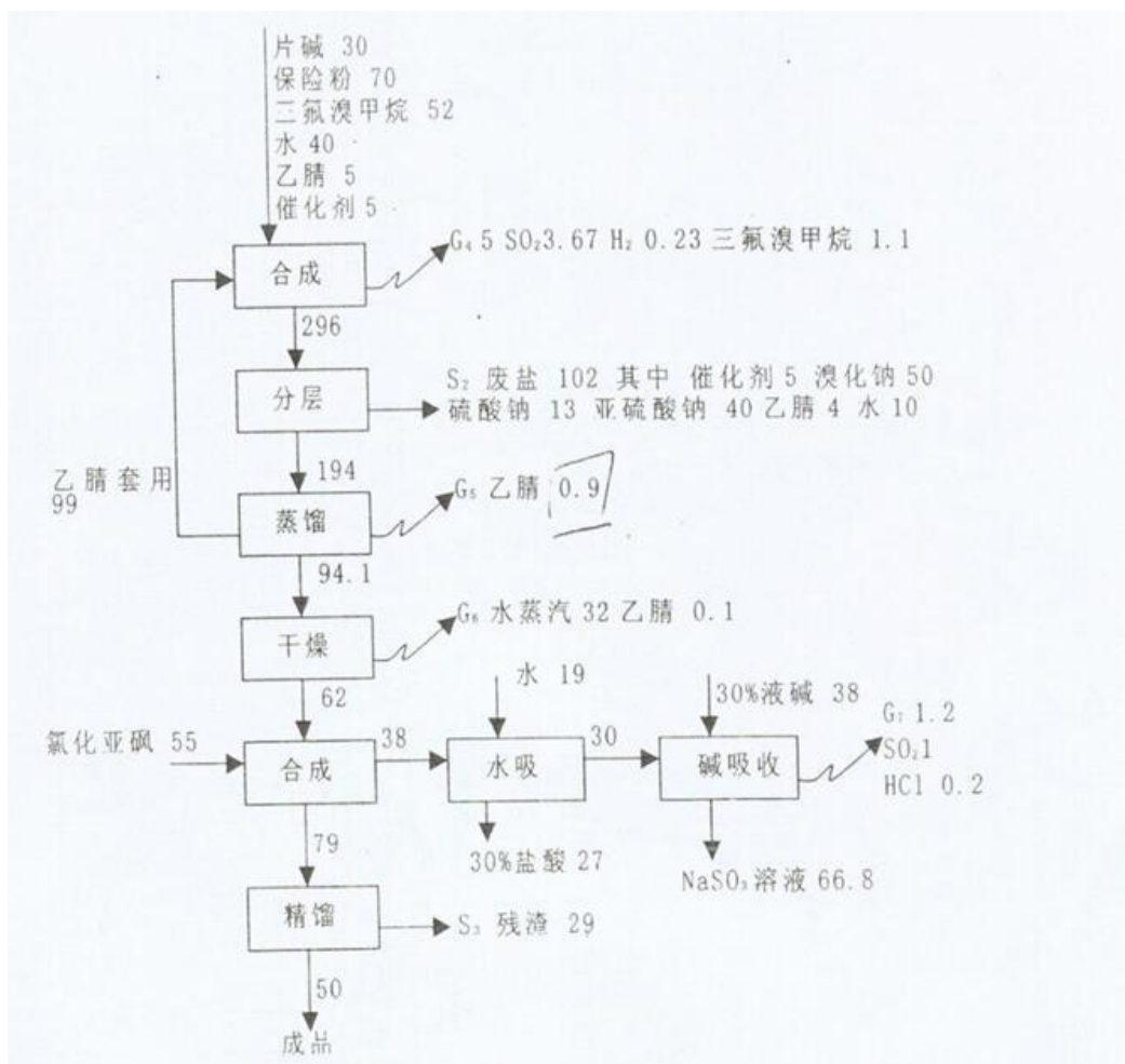
图 2.4-6 三氟甲基亚硫酸氯生产工艺流程图
