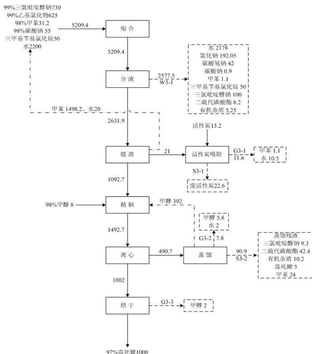
图 2.4-9 毒死蜱原药生产工艺流程图
