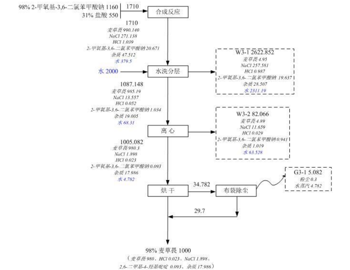
图 2.4-22 麦草畏生产工艺流程图
