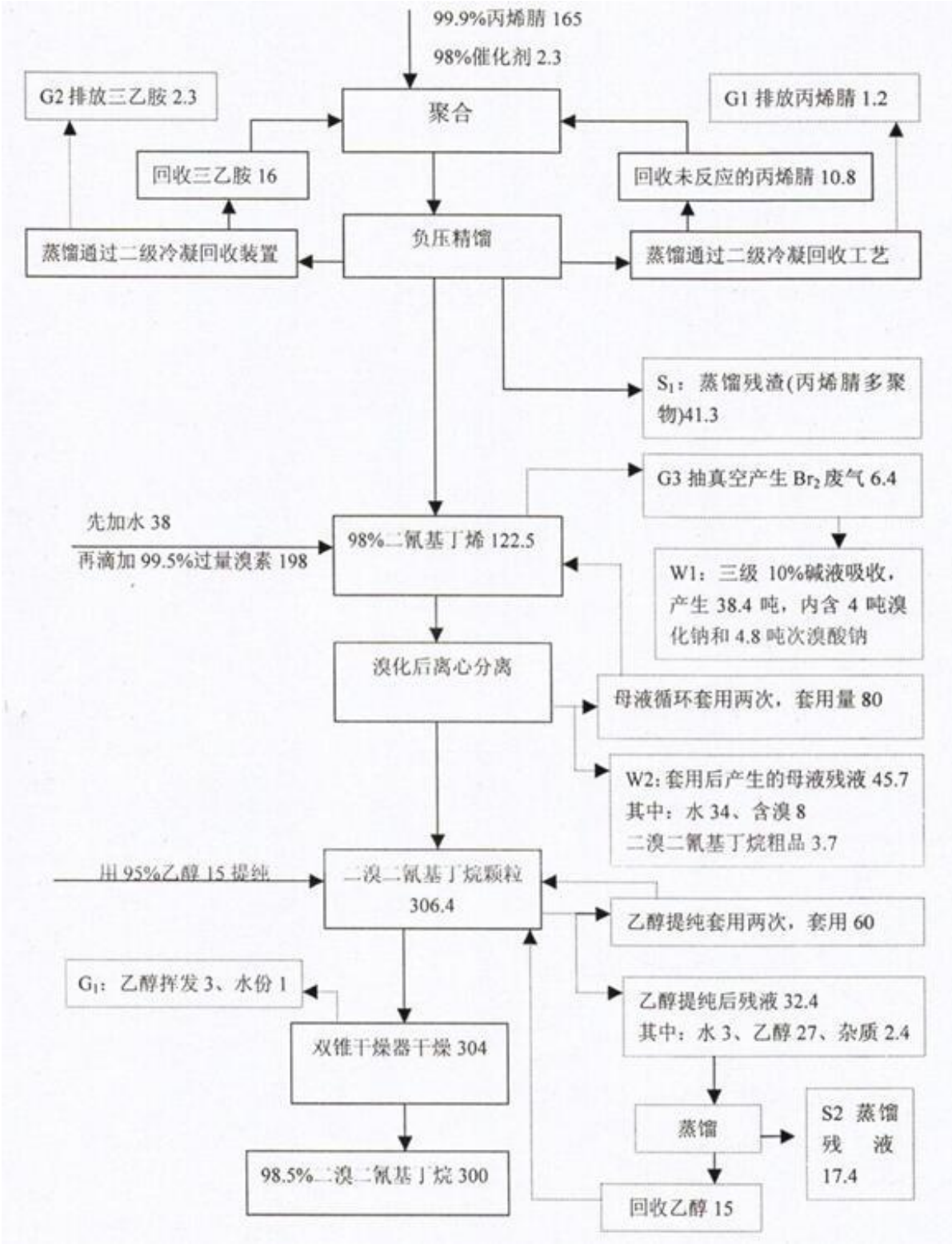
图 2.4-1 二溴二氰基丁烷生产工艺流程图
