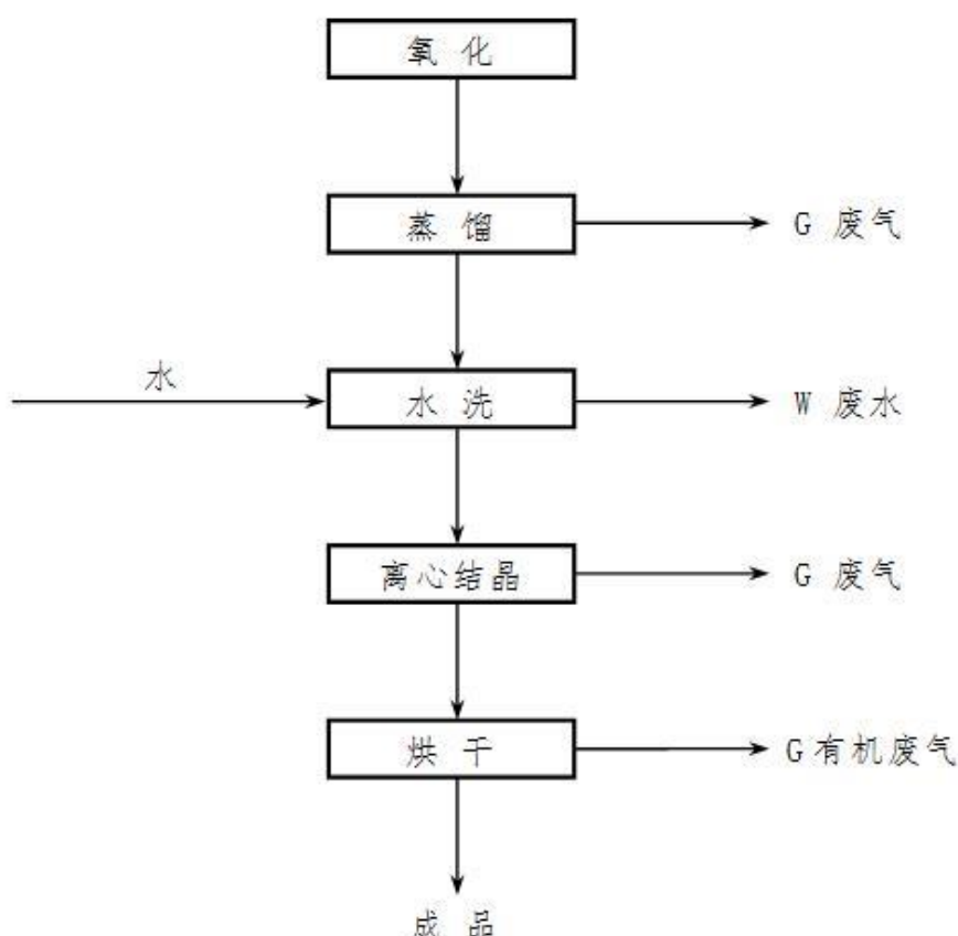
图 2.4-18 乙虫腈生产工艺流程图
