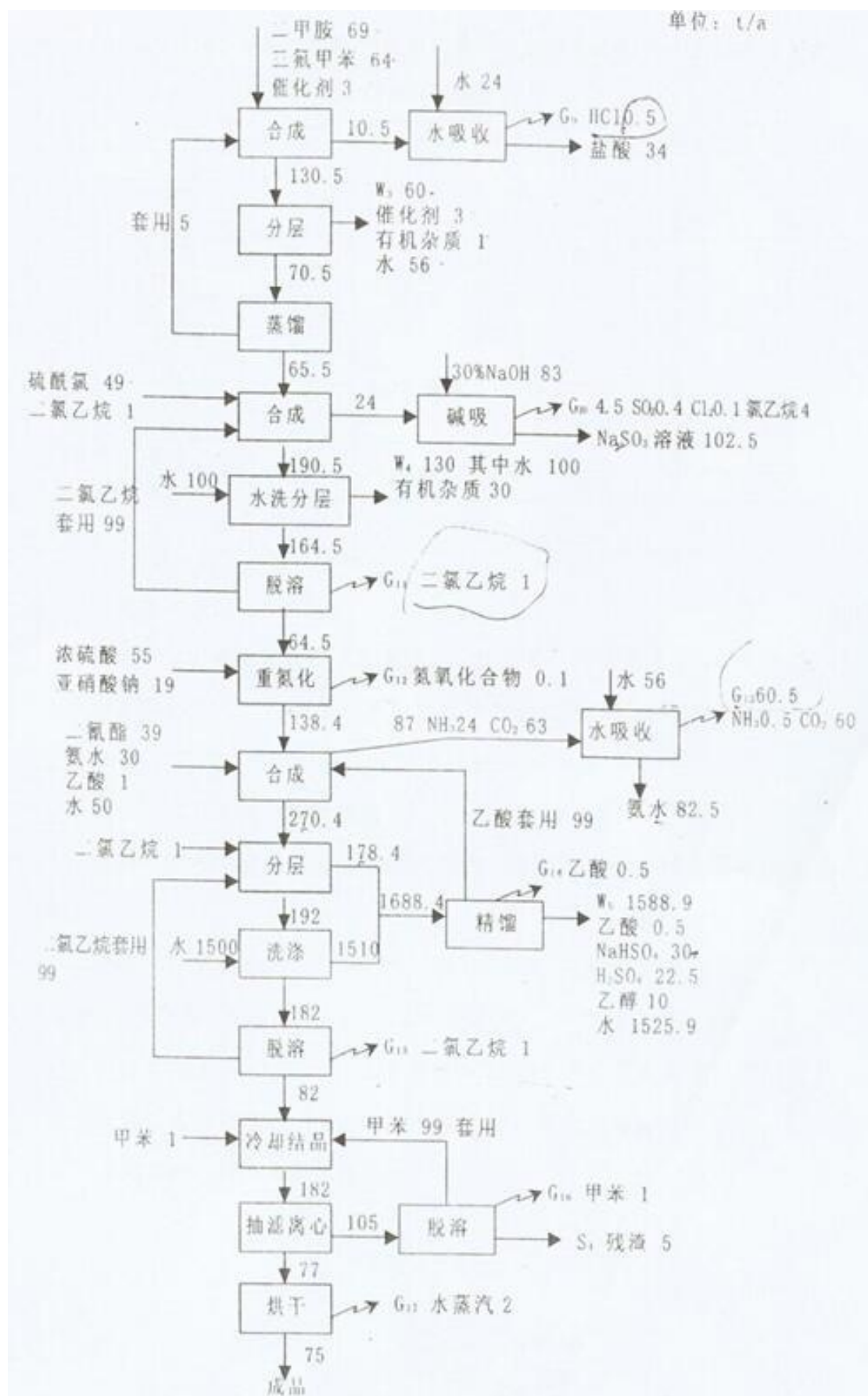
图 2.4-5 5-氨基-3-氟基-1-(2,6-二氯-4-三氟甲基苯基)生产工艺流程图
