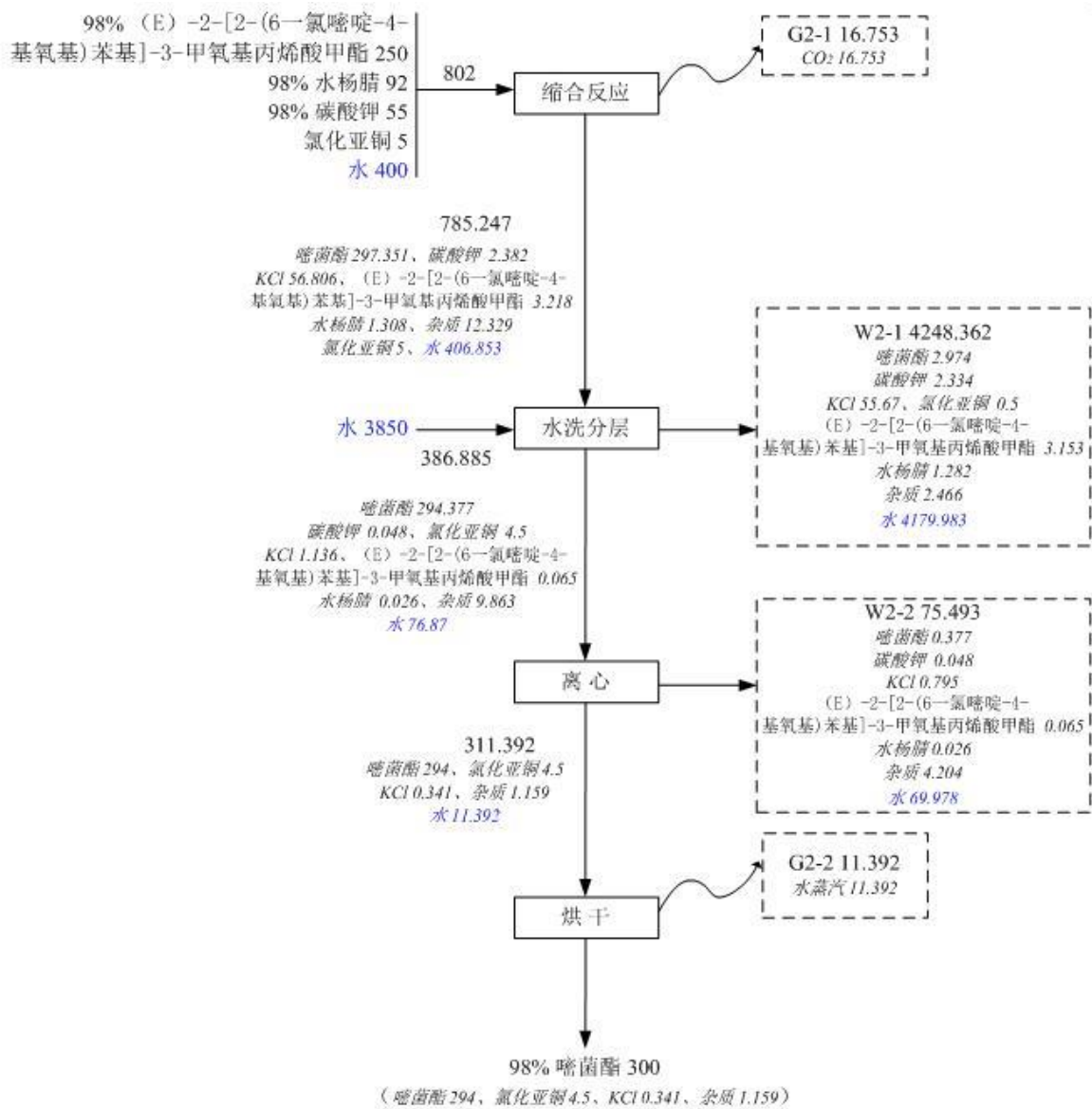
图 2.4-21 嘧菌酯生产工艺流程图
