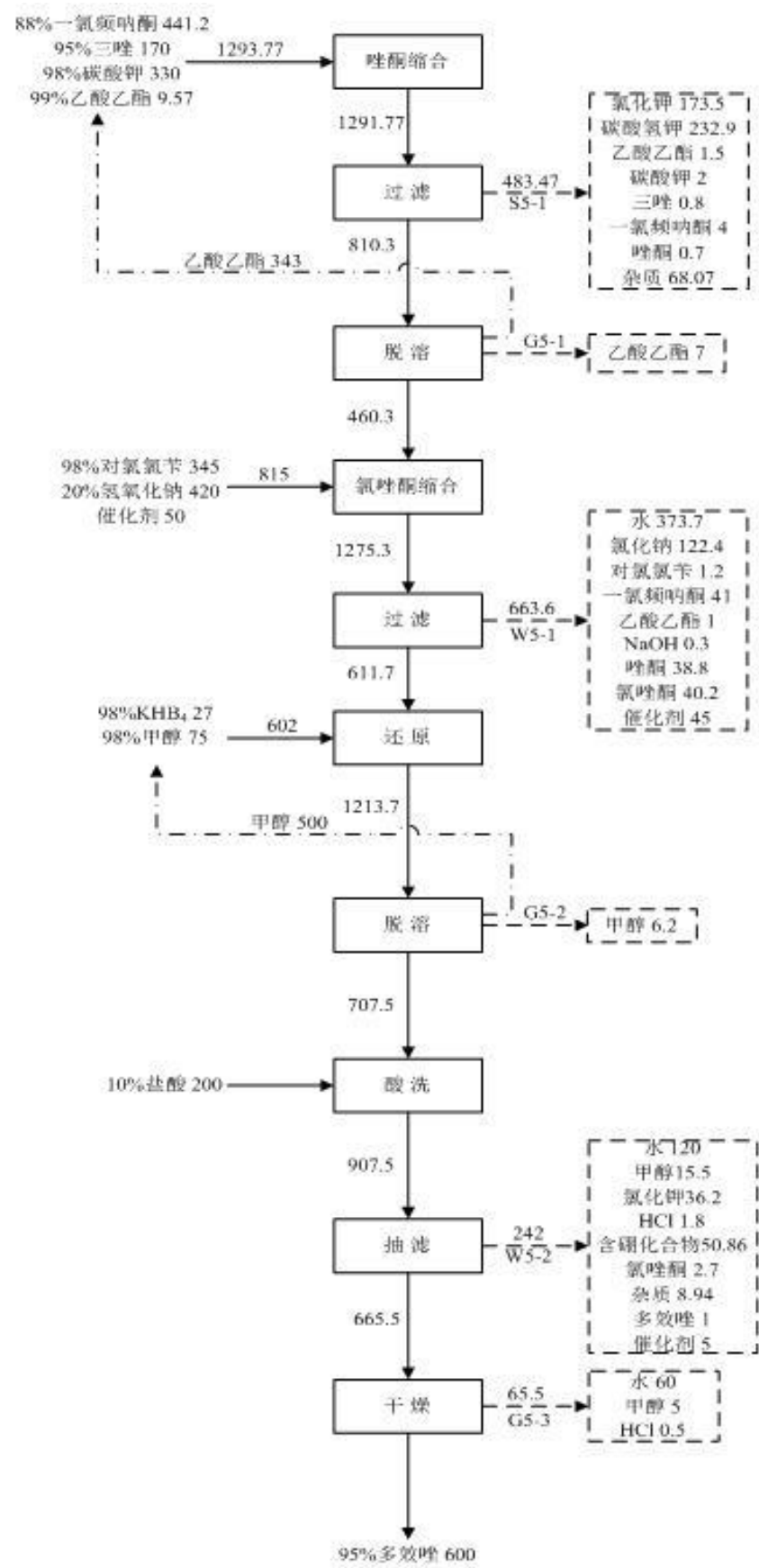
图 2.4-12 多效唑原药生产工艺流程图
