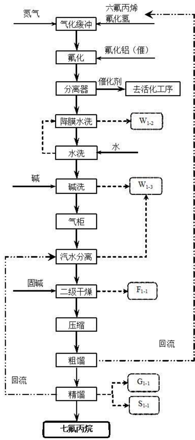
图 2.4-15 七氟丙烷生产工艺流程图
