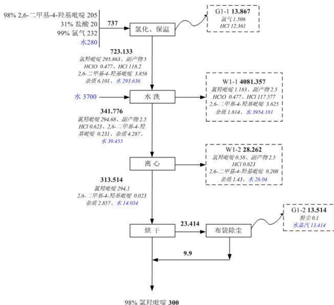
图 2.4-20 氯羟吡啶生产工艺流程图
