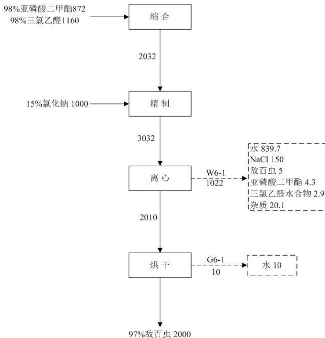
图 2.4-10 敌百虫原药生产工艺流程图
