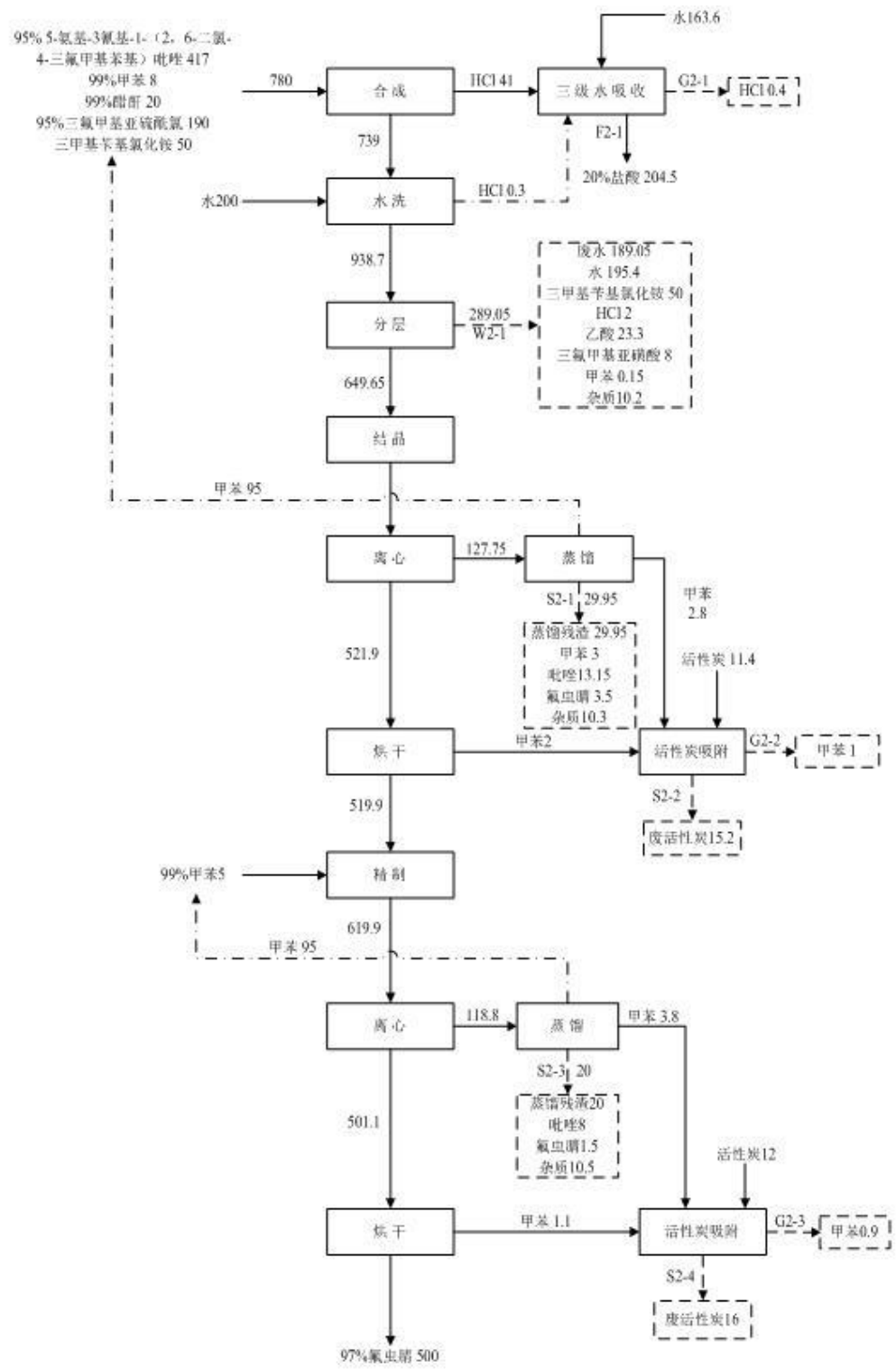
图 2.4-8 氟虫腓原药生产工艺流程图
