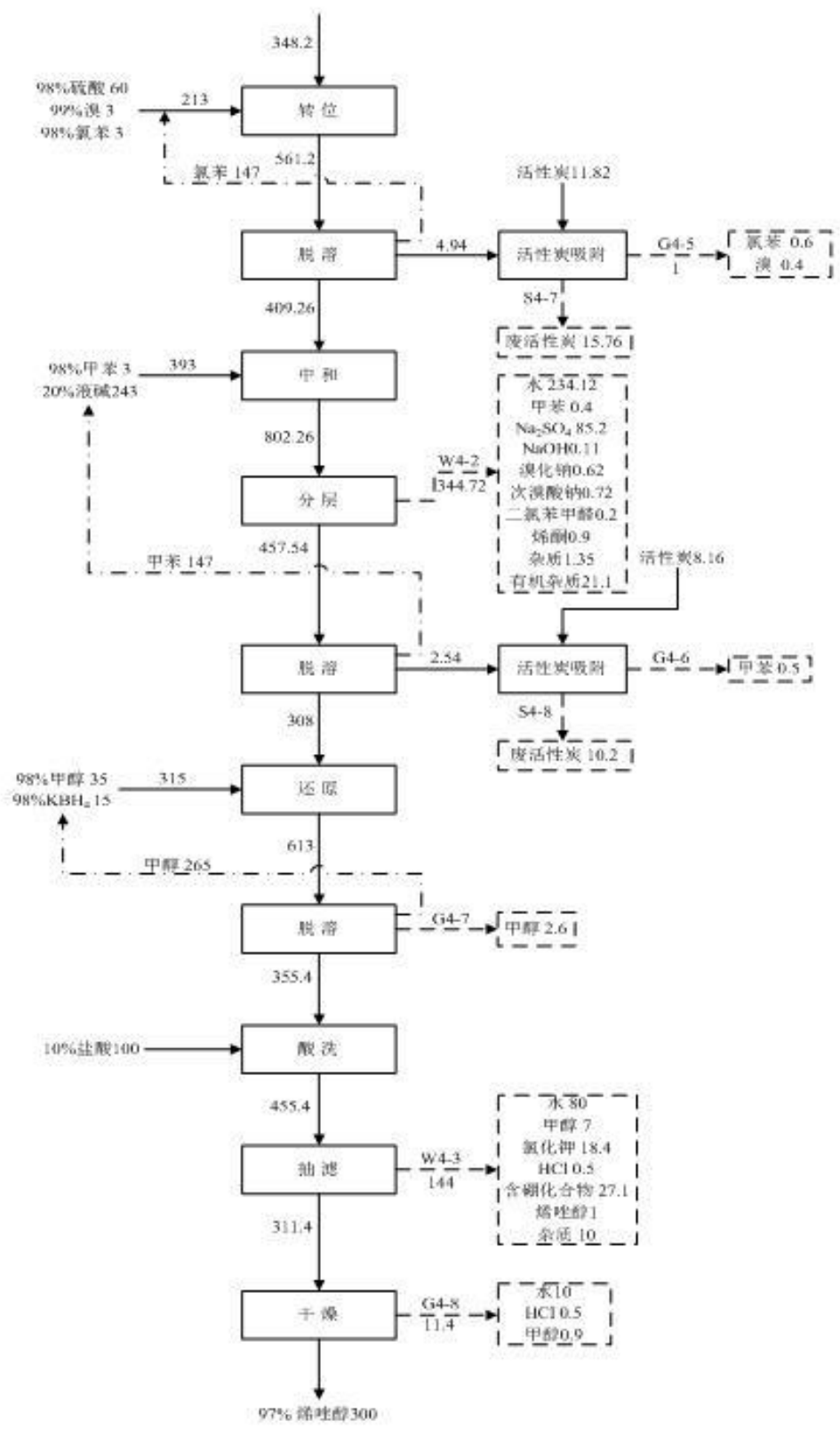
图 2.4-11 烯唑醇原药生产工艺流程图
