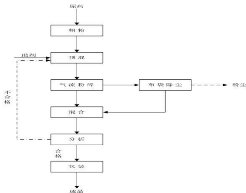
图 2.4-14 粉剂生产工艺流程图
