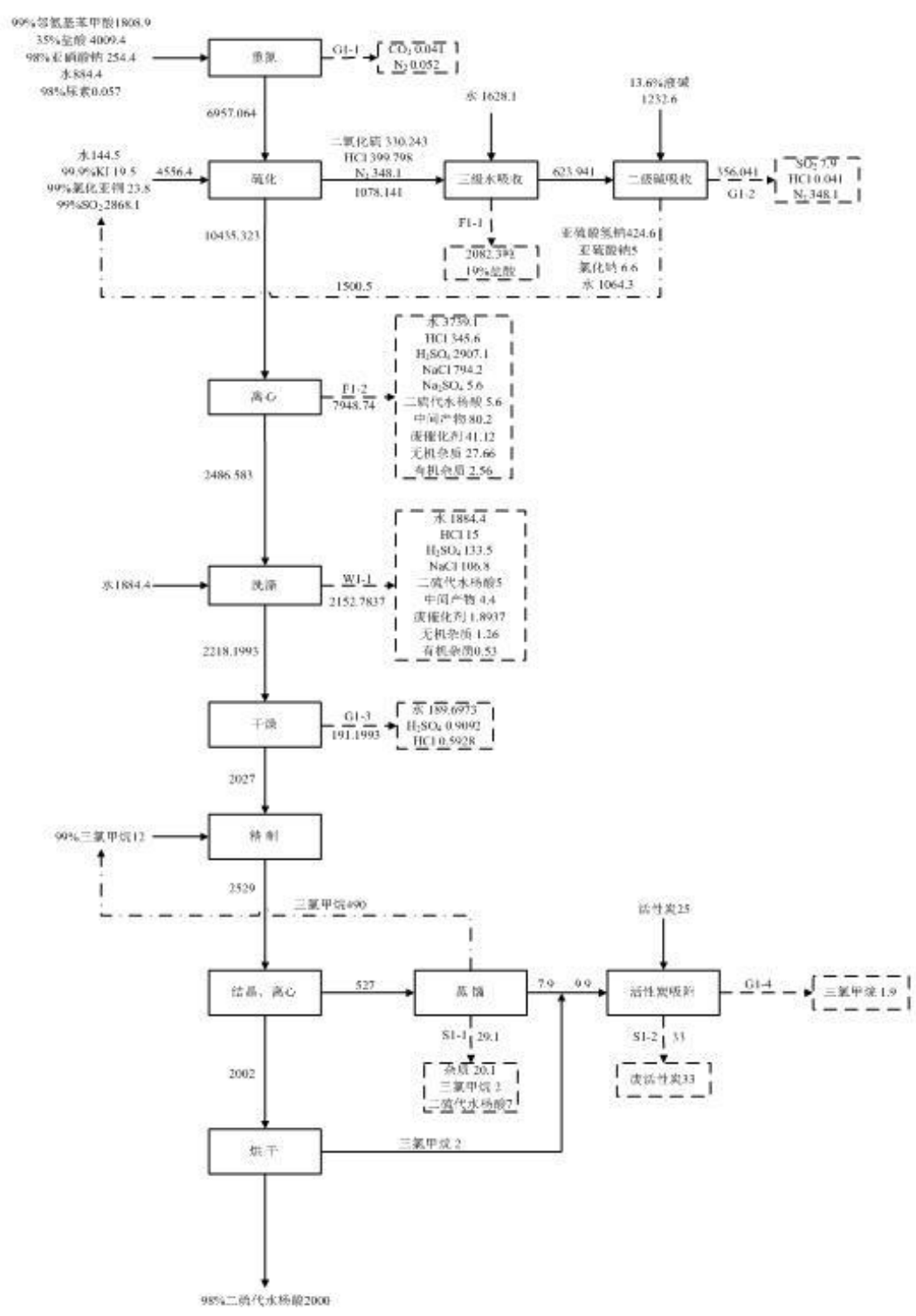
图 2.4-7 二磺代水杨酸生产工艺流程图
