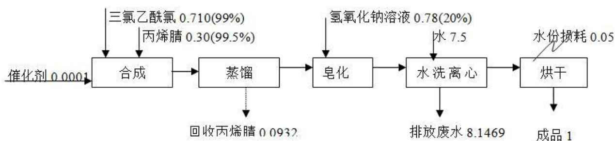
图 2.4-3 3,5,6-三氯吡啶醇钠生产工艺流程图
