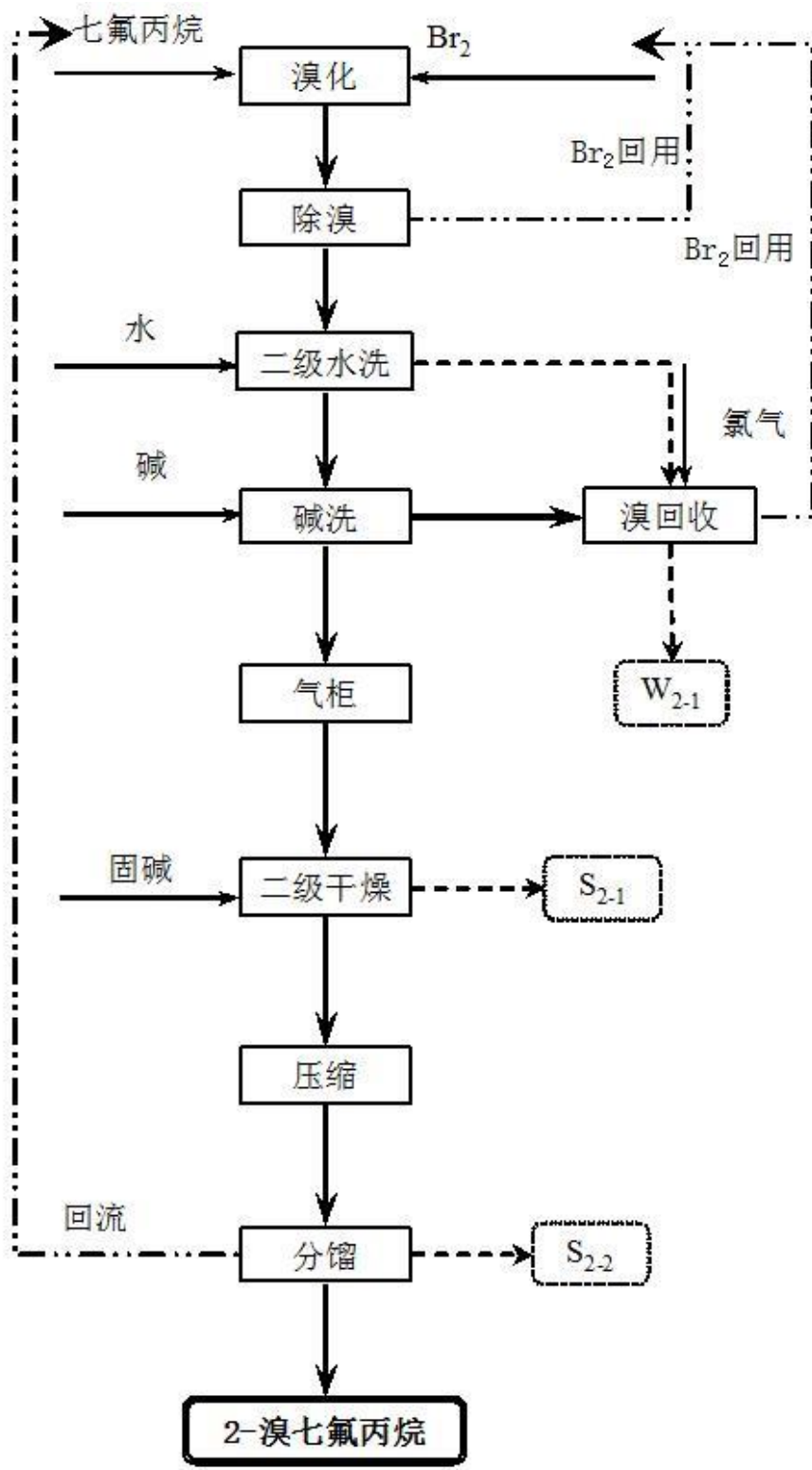
图 2.4-16 2-溴七氟丙烷生产工艺流程图
