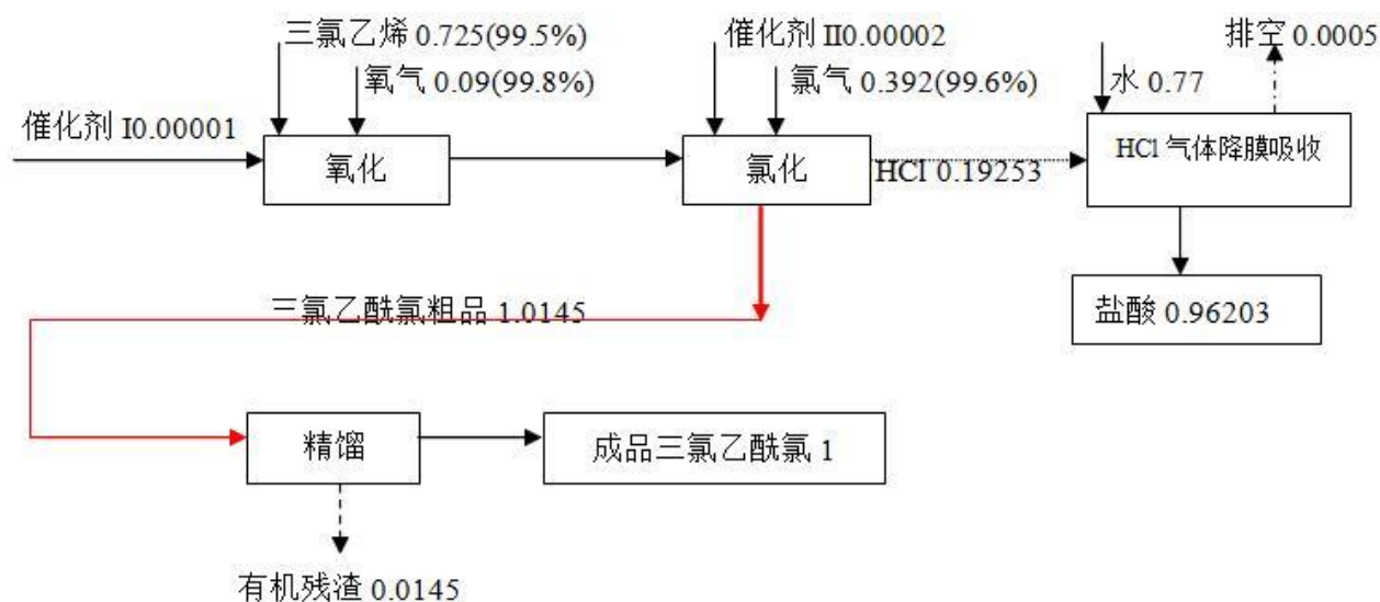
图 2.4-2 三氯乙酐氯生产工艺流程图
