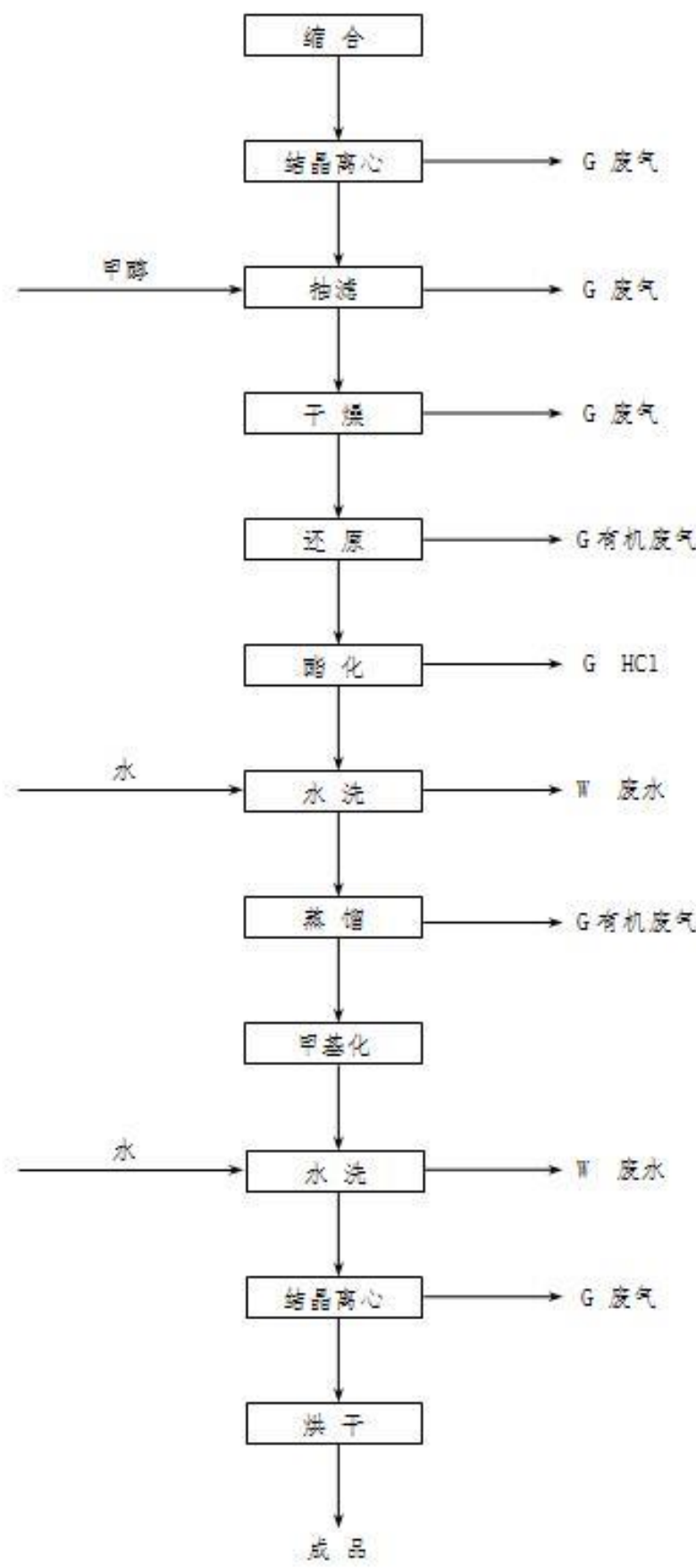
图 2.4-17 吡唑醚菌酯生产工艺流程图
