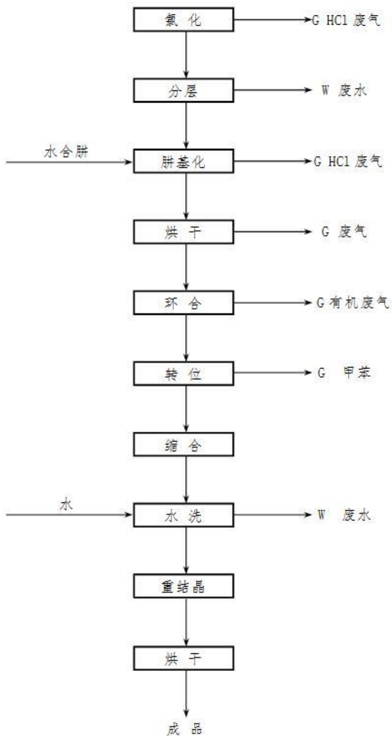
图 2.4-19 五氟磺草胺生产工艺流程图
