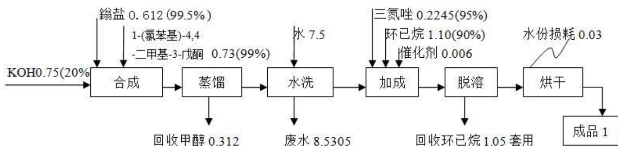
图 2.4-4 氯苯三唑戊醇生产工艺流程图
