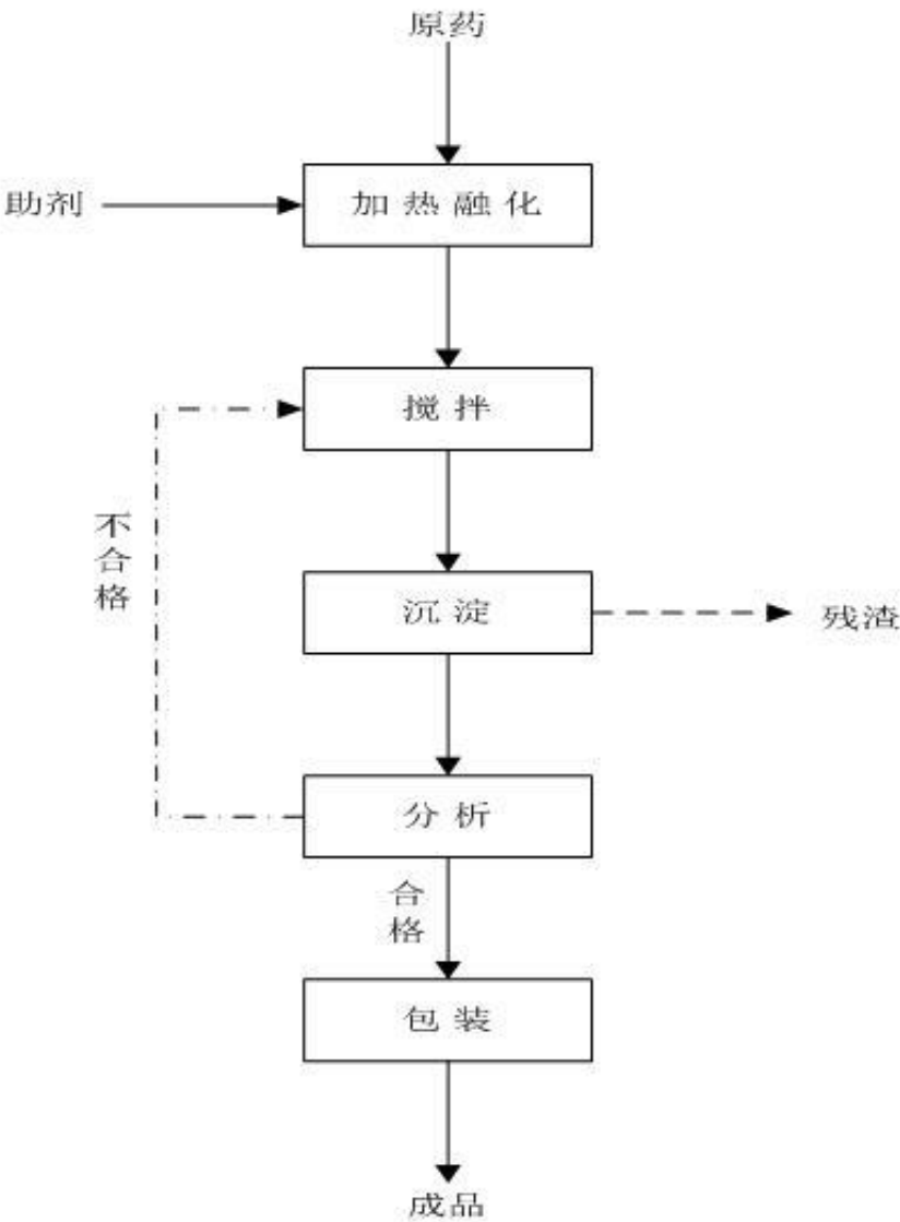
图 2.4-13 液体制剂生产工艺流程图
